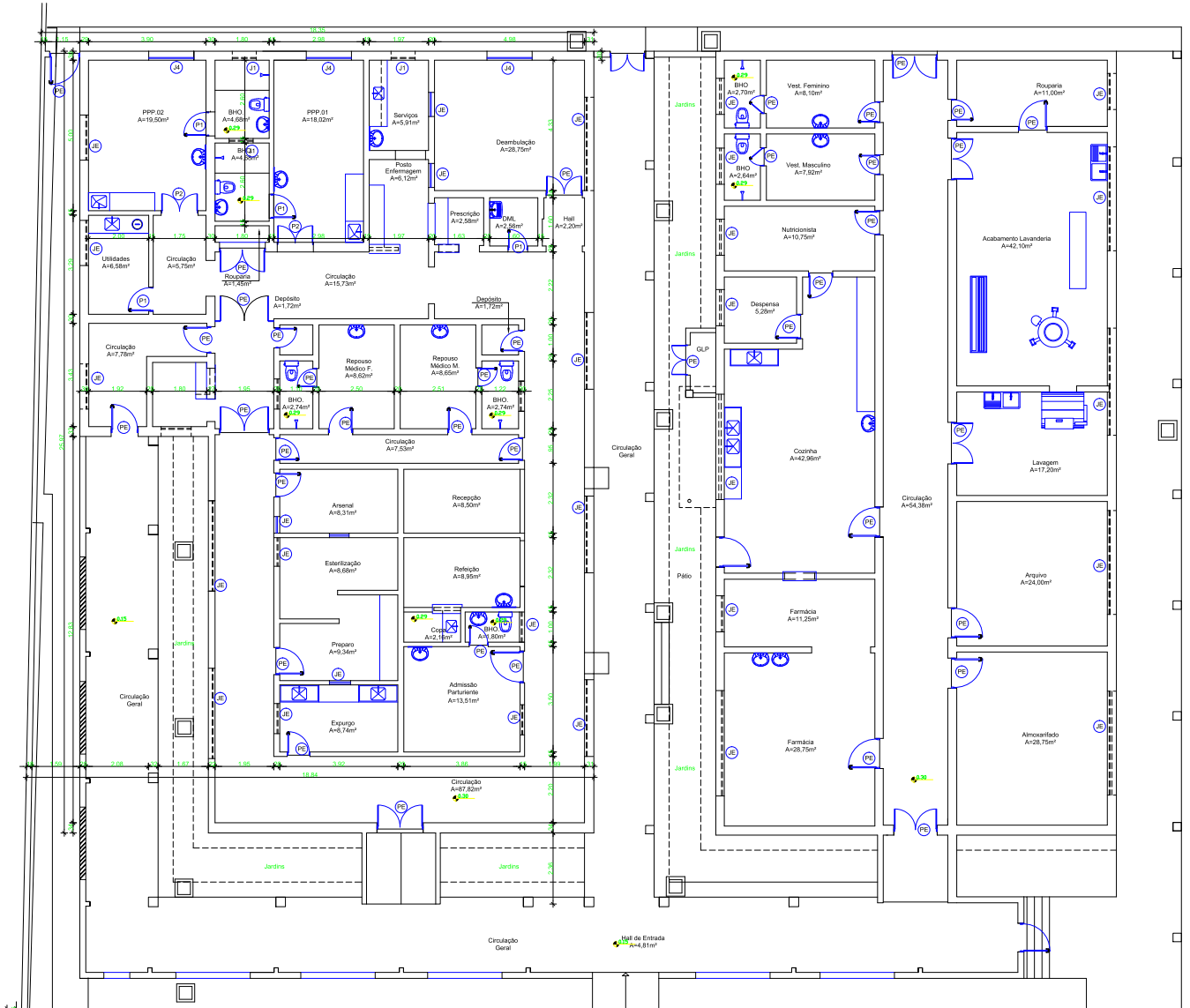
02 Planta Especificações - Setor 02 ESC. 1/75
