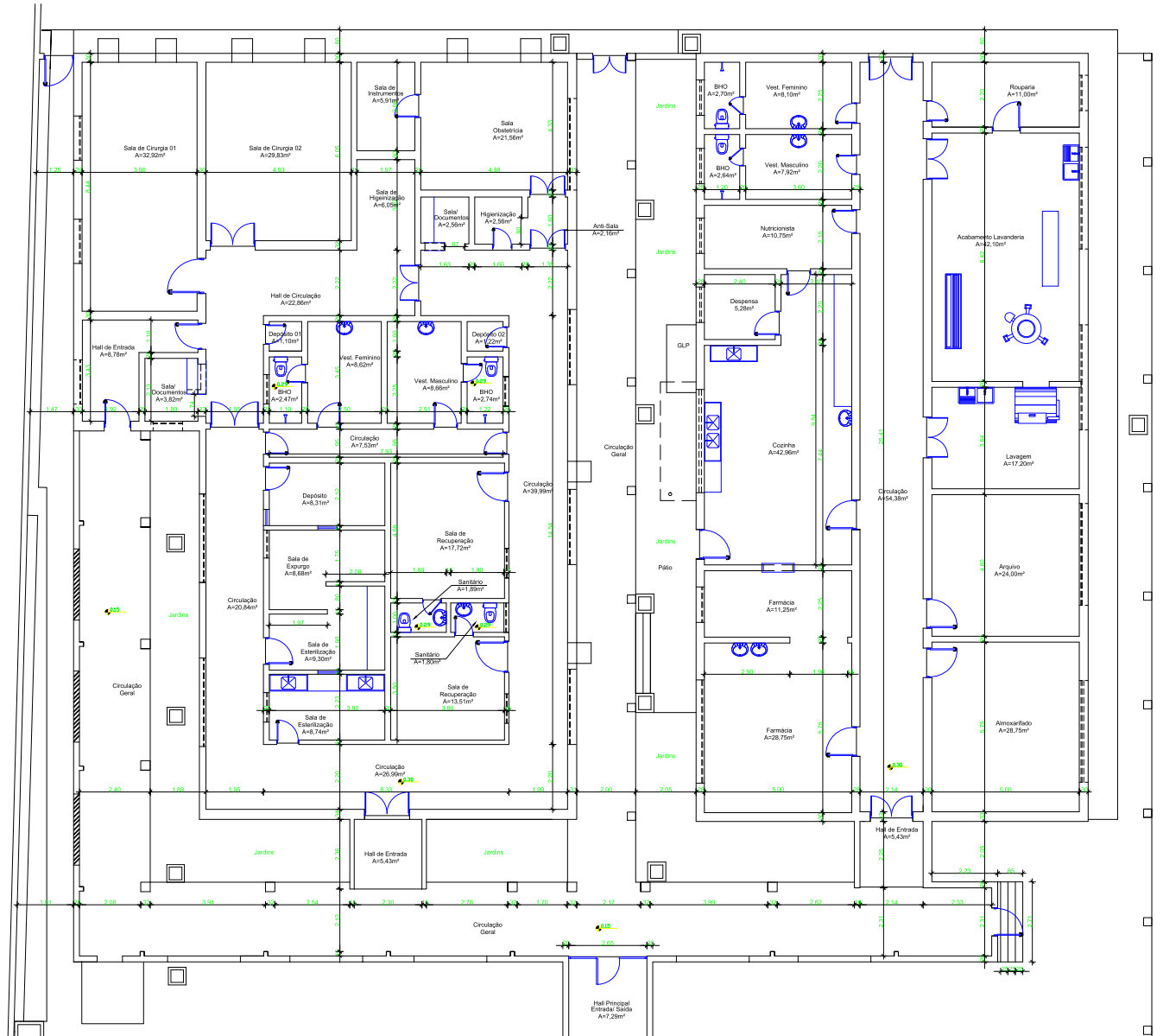
01 Planta Existente - Setor 02 ESC. 1/75
