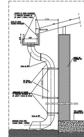
DETALHE - 02 DA DESCIDA DE ÁGUAS PLUVIAIS
