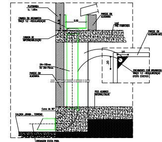
DETALHE - 03 DA DESCIDA DE ÁGUAS PLUVIAIS
