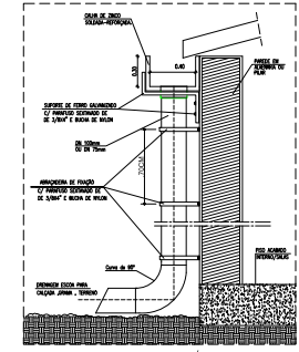
DETALHE - 01 DA DESCIDA DE ÁGUAS PLUVIAIS
