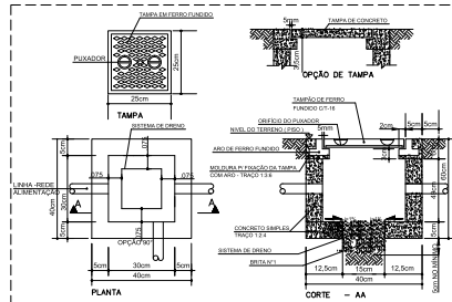
03 DETALHE - CAIXA DE PASSAGEM (001) 40X40X60CM SEM ESCALA
