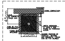
02 DETALHE 04 - LEITO DE TUBO PVC SEM ESCALA
