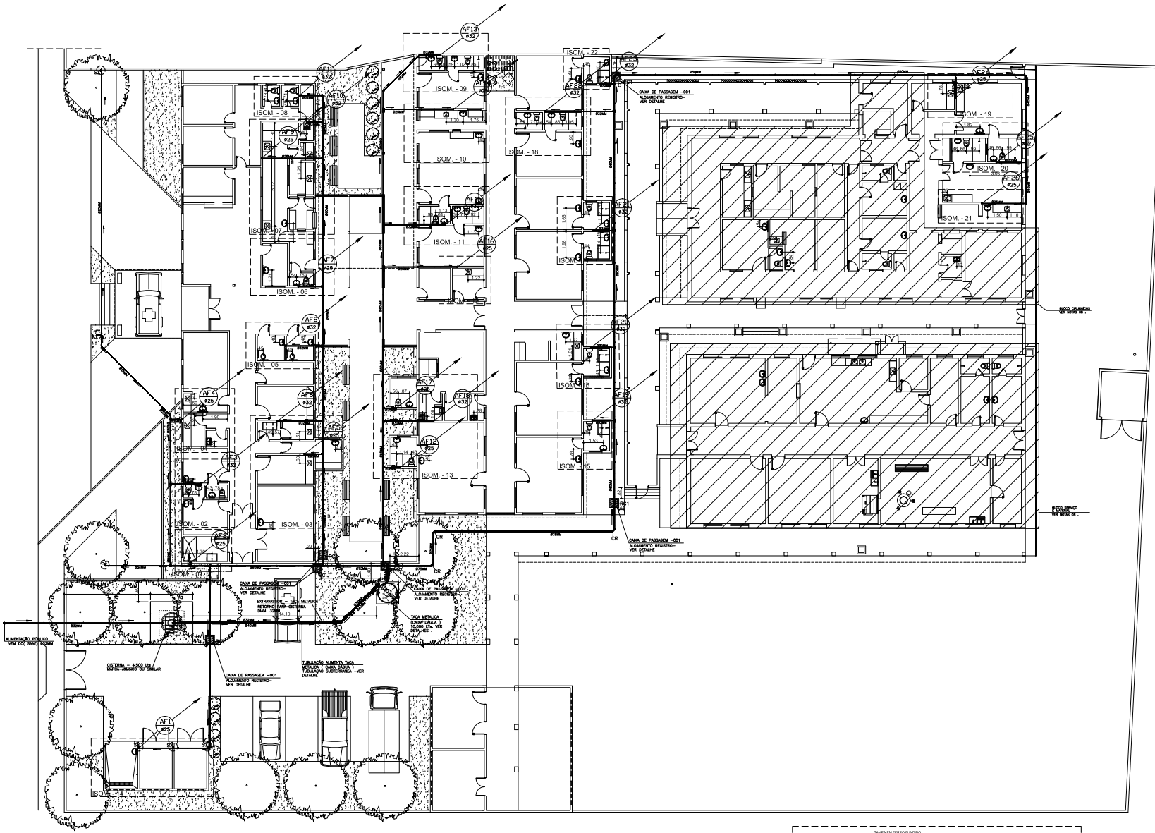
01 PLANTA BAIXA - REDE DE ÁGUA ESCALA 1:100
