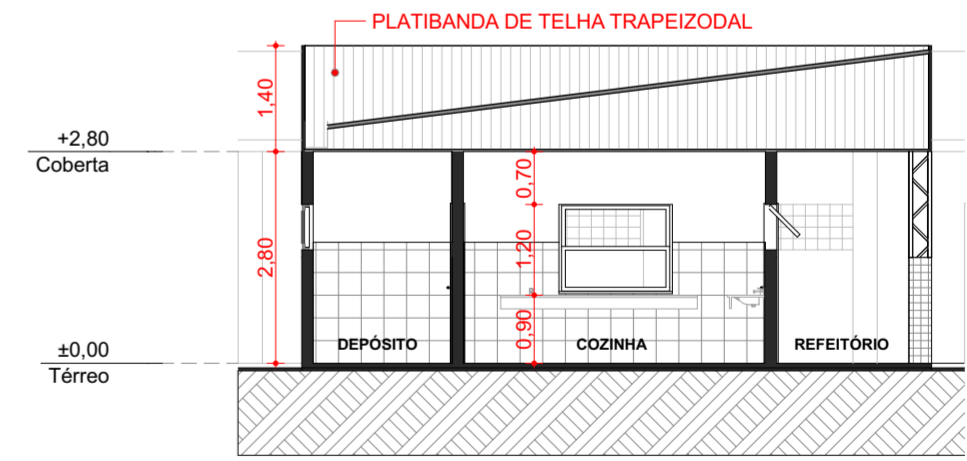
3 CORTE B ESC.: 1:100
