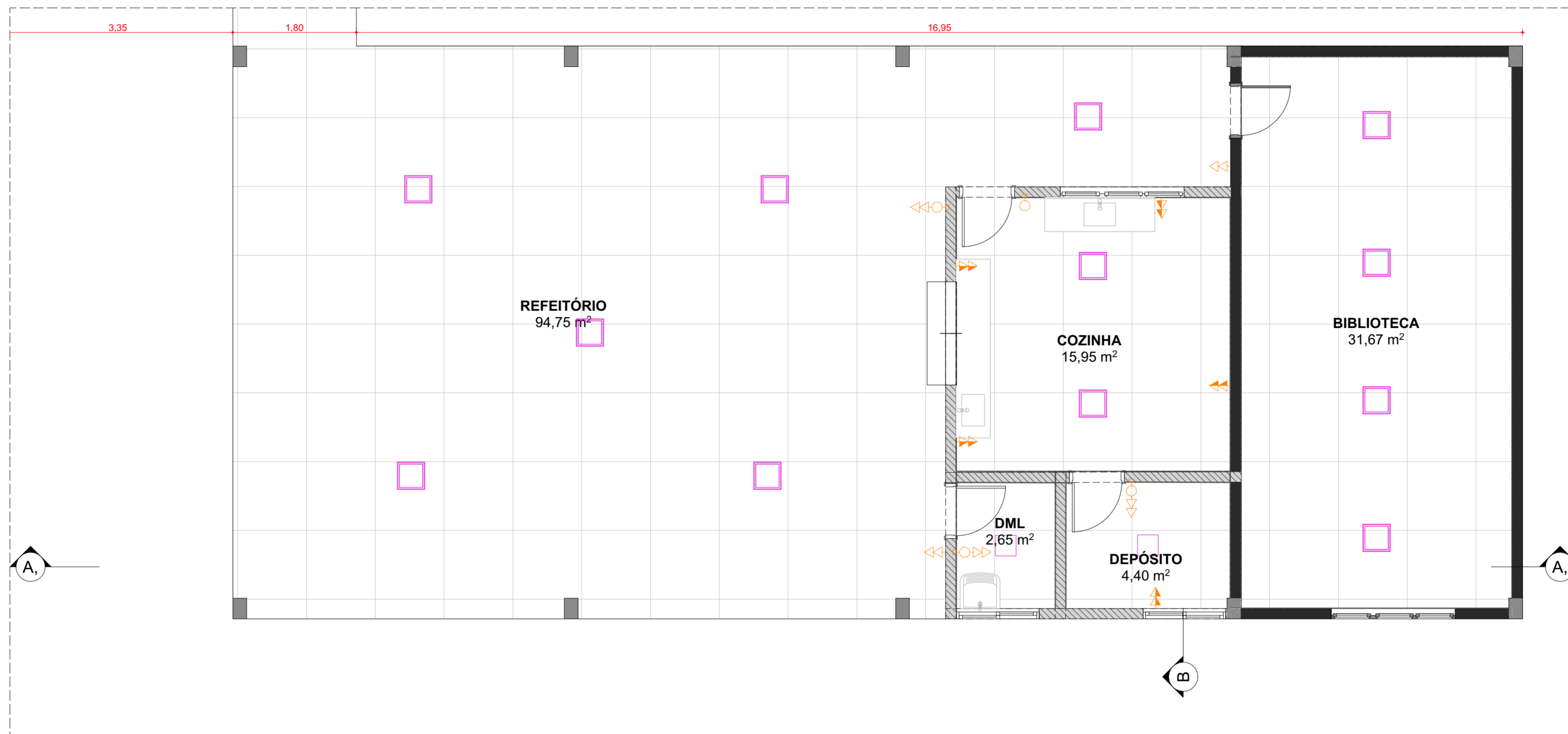
1 PLANTA LUMINOTÉCNICA E ELÉTRICA ESC.: 1:50
