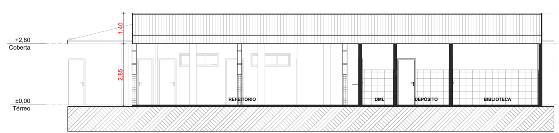
2 CORTE A ESC.: 1:100
