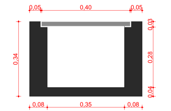
4 CORTE A ESC.: 1:10
