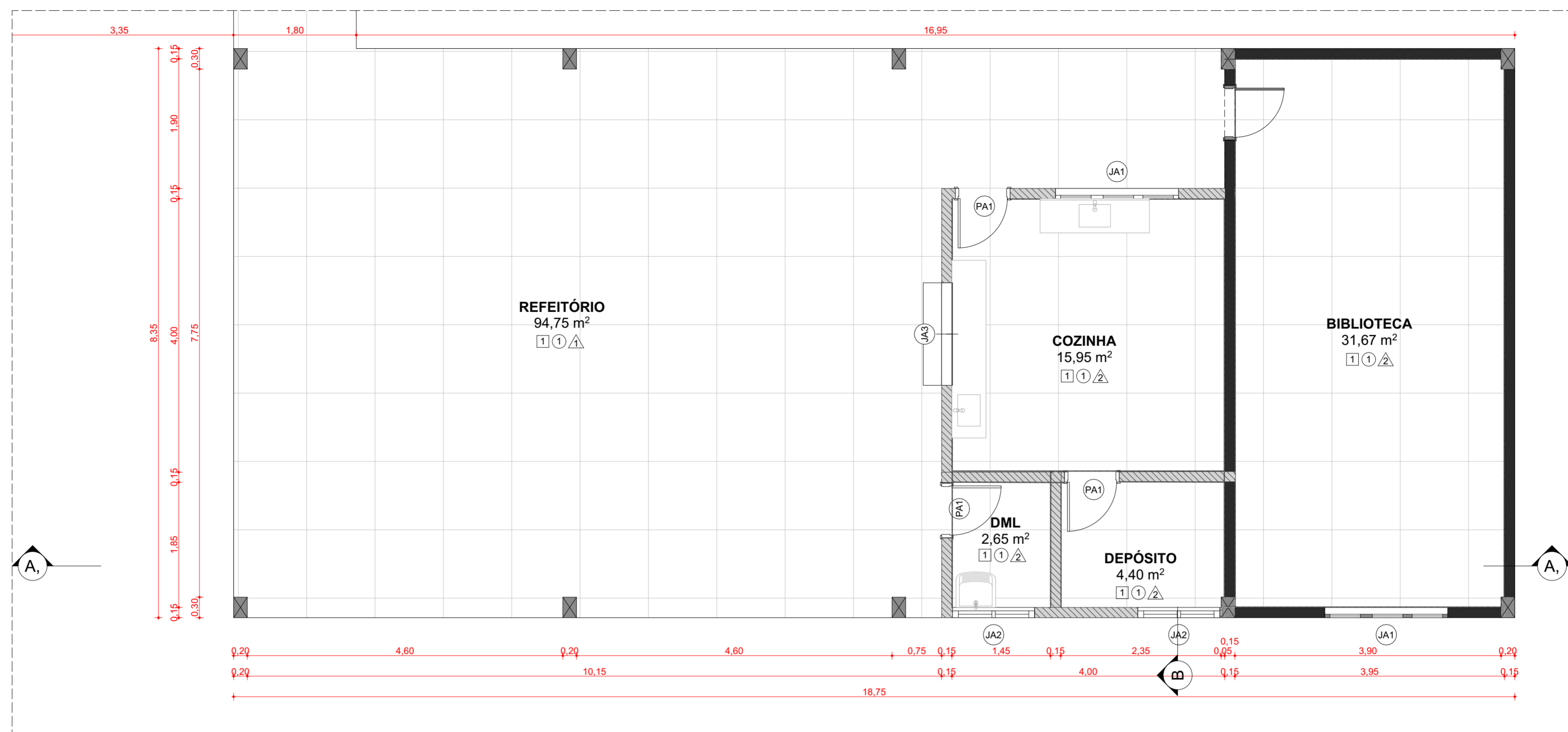
1 PLANTA DE REFORMA ESC.: 1:50
