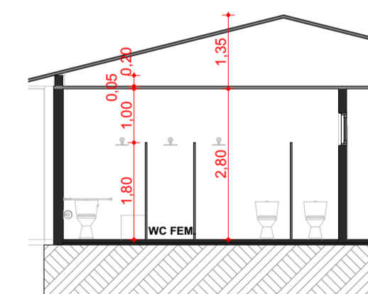
4 CORTE C ESC.: 1:100
