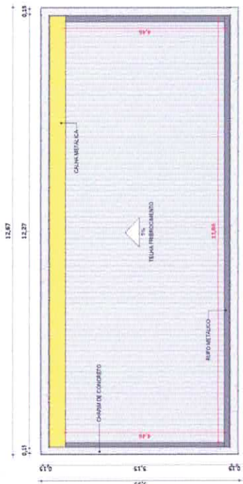
1 PLANTA DE COBERTURA Escala: 1:50
